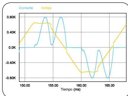
FORMAS DE ONDA DE ENTRADA
