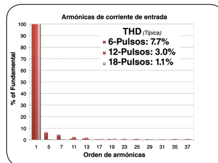
ESPECTRO DE ARMÓNICAS DE ENTRADA
